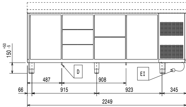
Zij aanzicht
